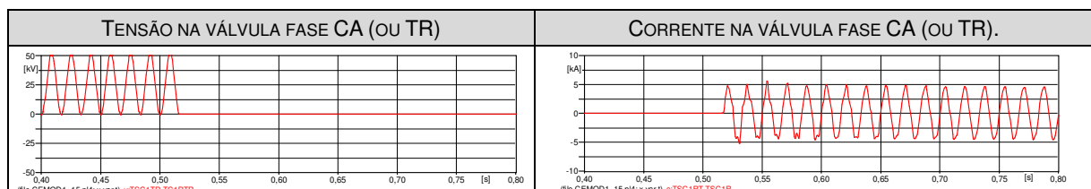
FIGURA 6 – Formas de onda da tensão e corrente na válvula com a energização do TSC com o capacitor previamente carregado.
