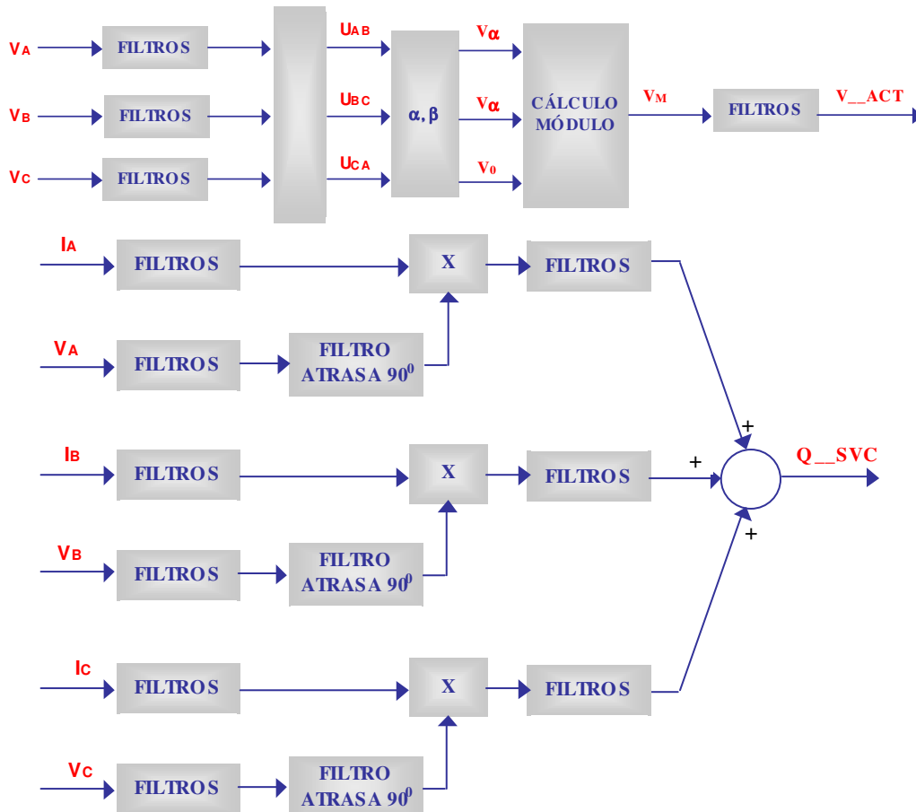
FIGURA 3 – Sistema de medição de tensão ( V\_ACT ).
