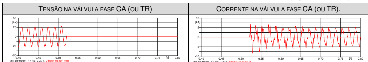
FIGURA 5 – Formas de onda da tensão e corrente na válvula com a energização do TSC com o capacitor previamente descarregado.
