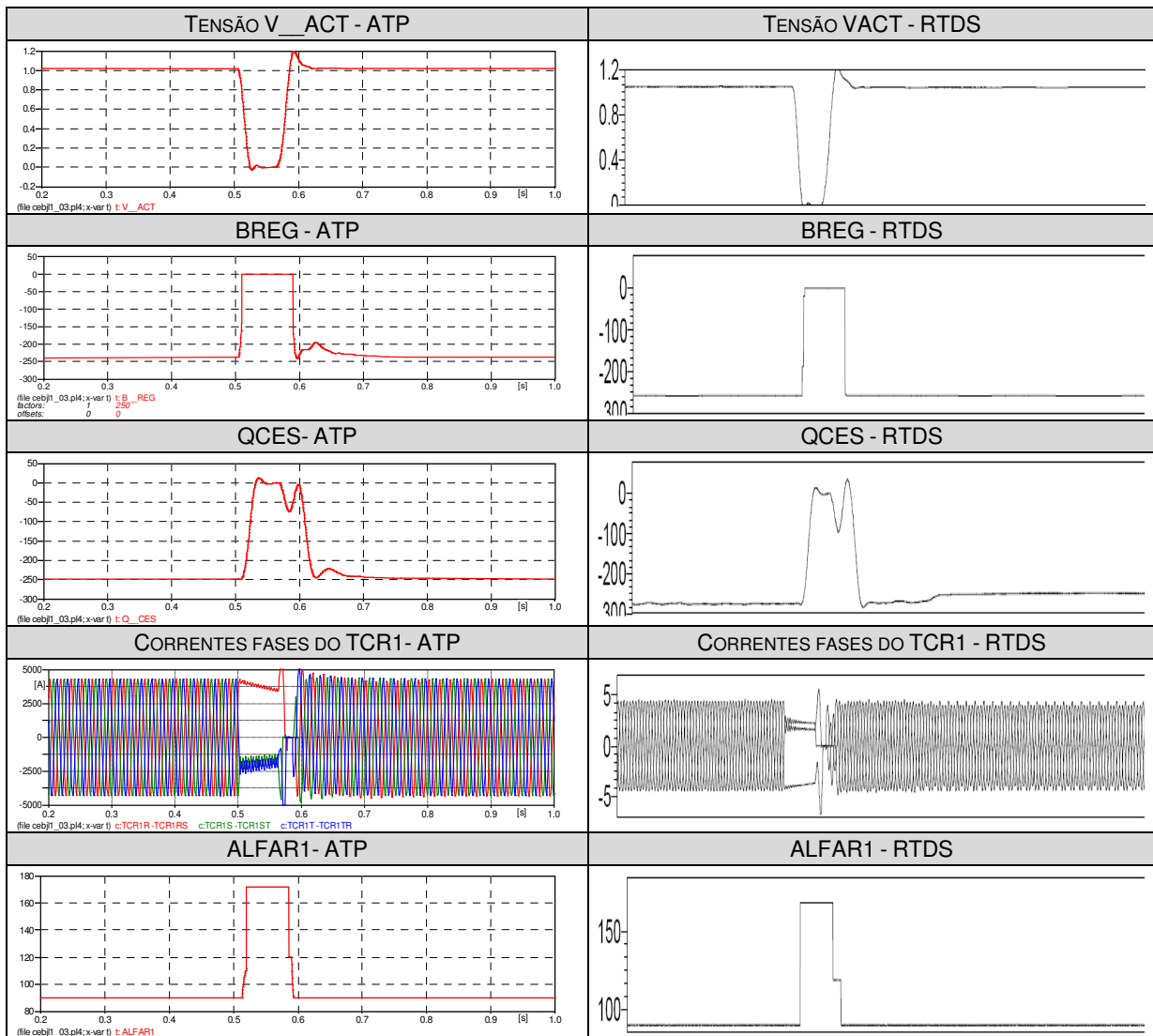
FIGURA 7 – Curto circuito trifásico Bom Jesus da Lapa 500kV.
