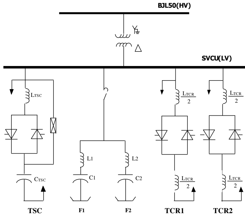
FIGURA 1 – Configuração básica do CE B JL.
